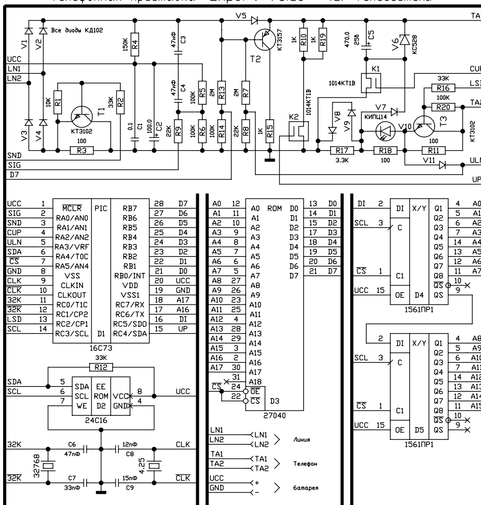
Телефонная приставка "Expert-Voice" (C) Телесистемы
