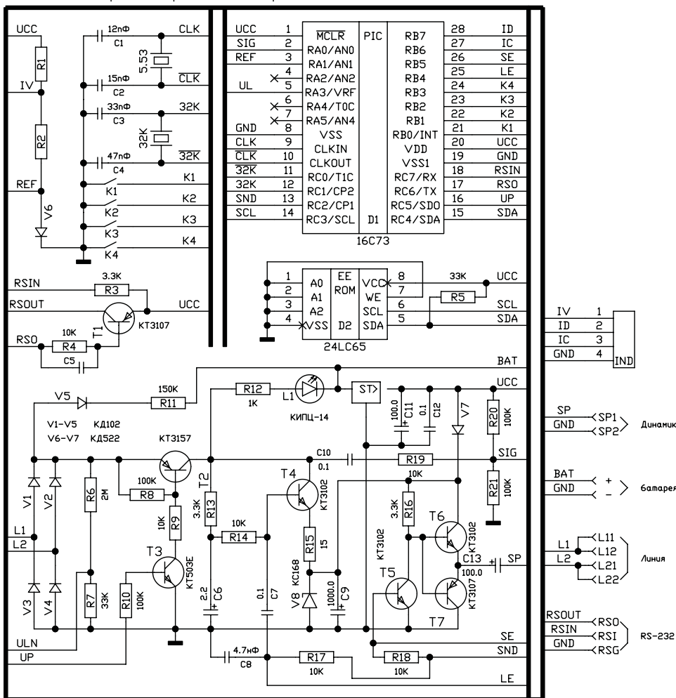
Телефонная приставка "Expert+" (C) Телесистемы
