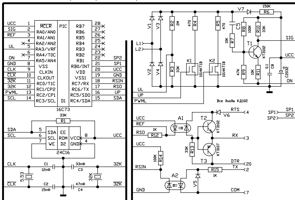
Телефонная приставка «Expert-PC» © Телесистемы
