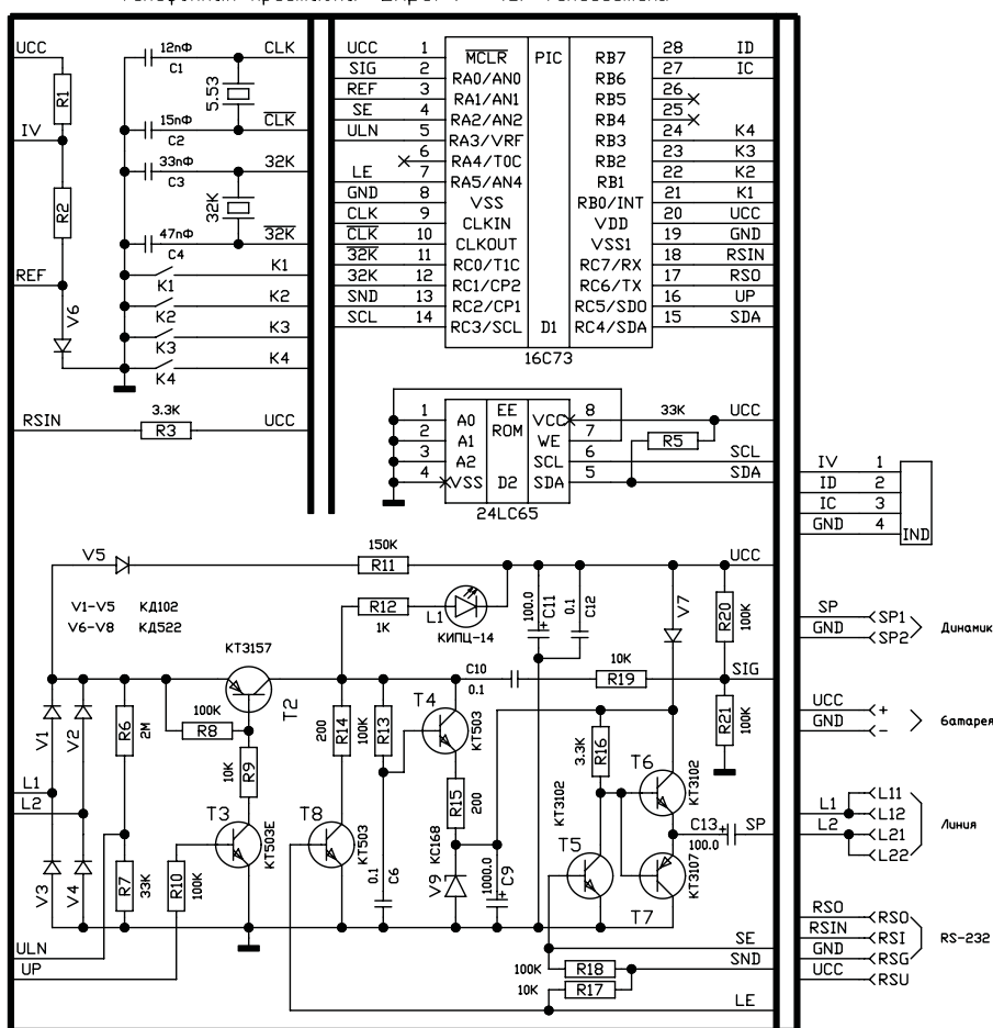
Телефонная приставка "Expert" (C) Телесистемы
